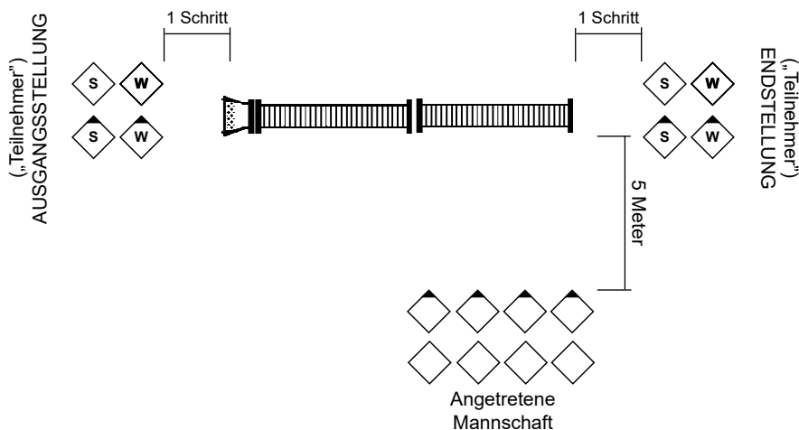
Skizze 6: Kuppeln von 2 Saugschläuchen
